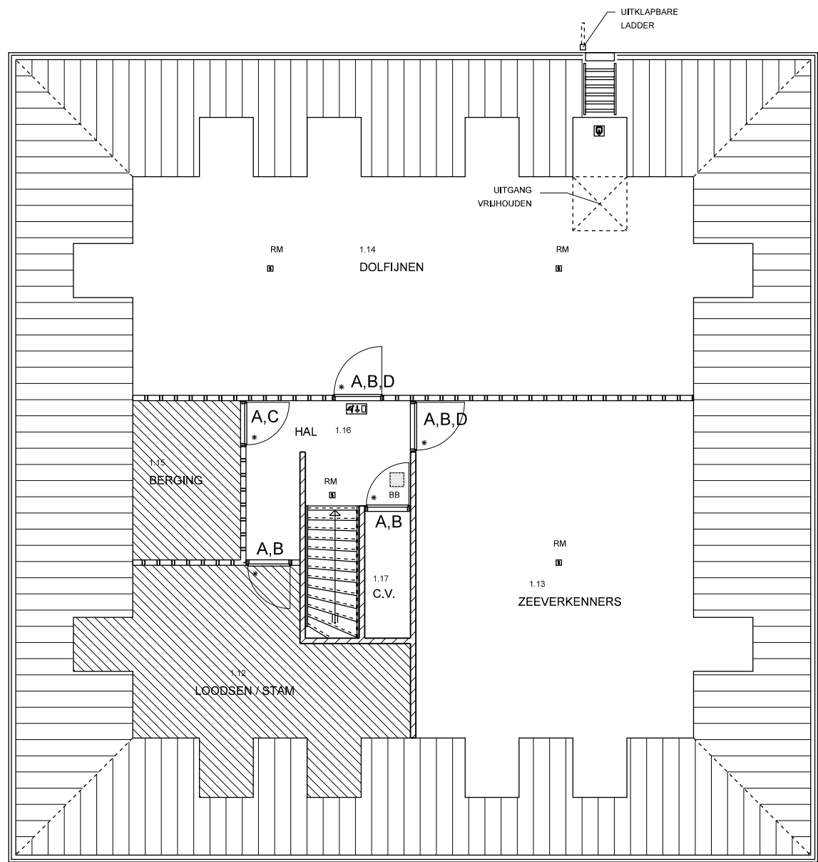
1ste Verdieping
